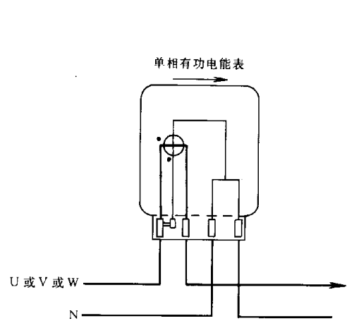
图 A.1 单相计量有功负荷直接接入方式
