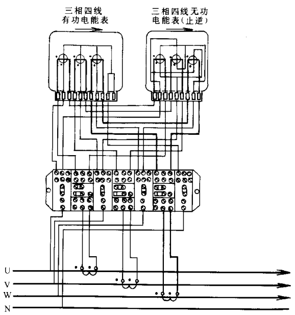
图 A.4 低压计量有功及无功电能电流分相接线方式
