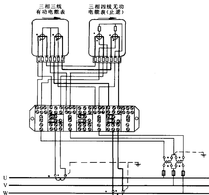
图 A.5 非有效接地系统高压计量有功及感性无功电能分相接线方式
