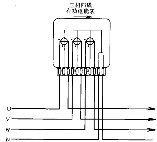
图 A.2 低压计量有功电能直接接入方式
