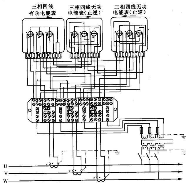
图 A.7 有效接地系统高压计量有功及感性、容性无功电能分相接线方式
