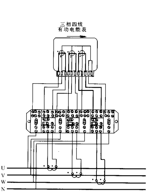
图 A.3 低压计量有功电能分相接线方式
