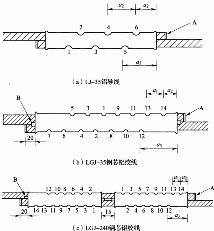
图 8.4.10 钳压管连接
